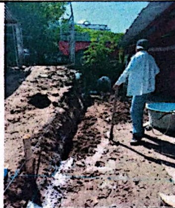
Foto 2: Sanjeado de las tres paredes del mejoramiento tipo pórtico.
